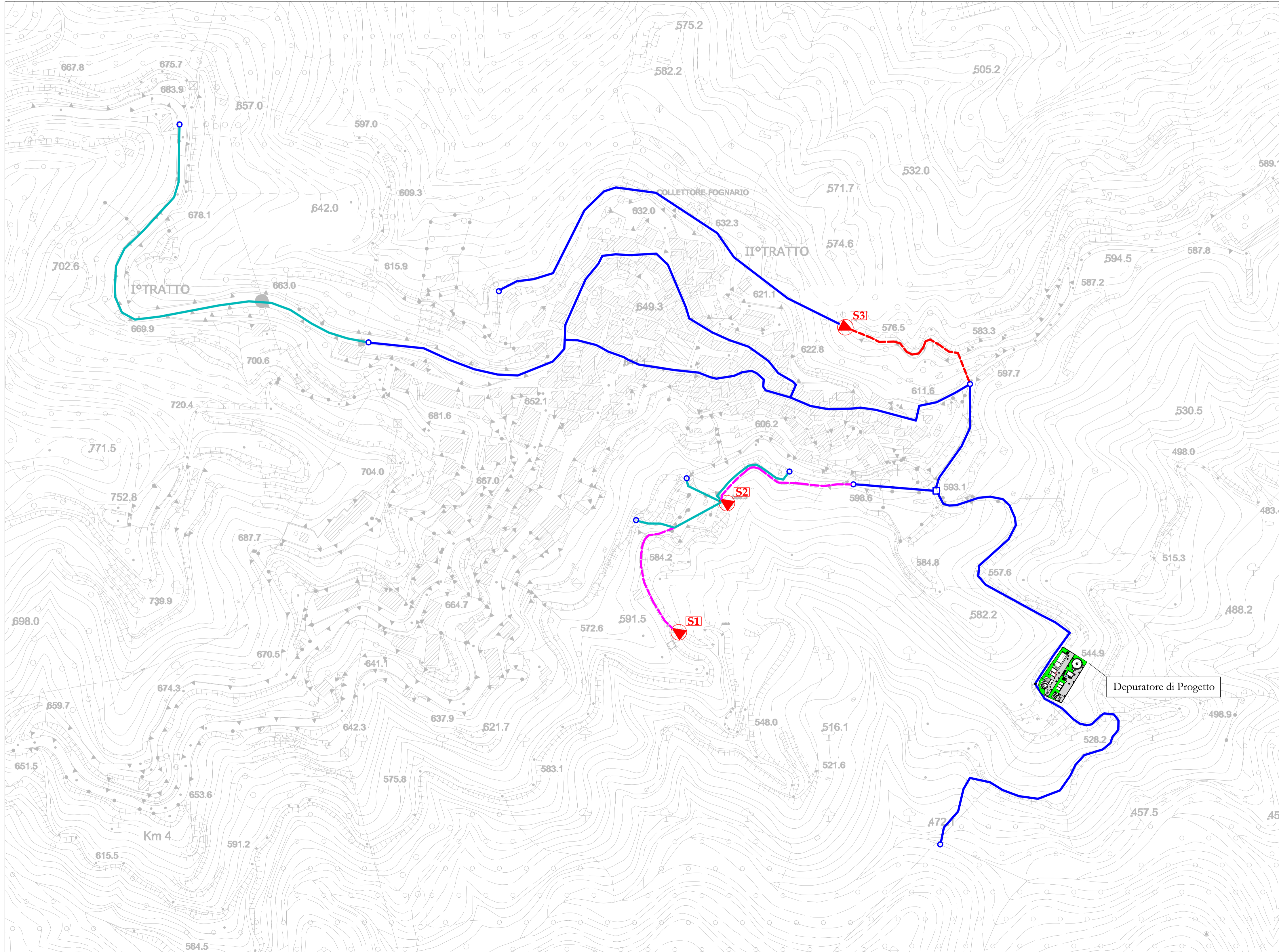
Planimetria Interventi di Progetto Pentone Centro
