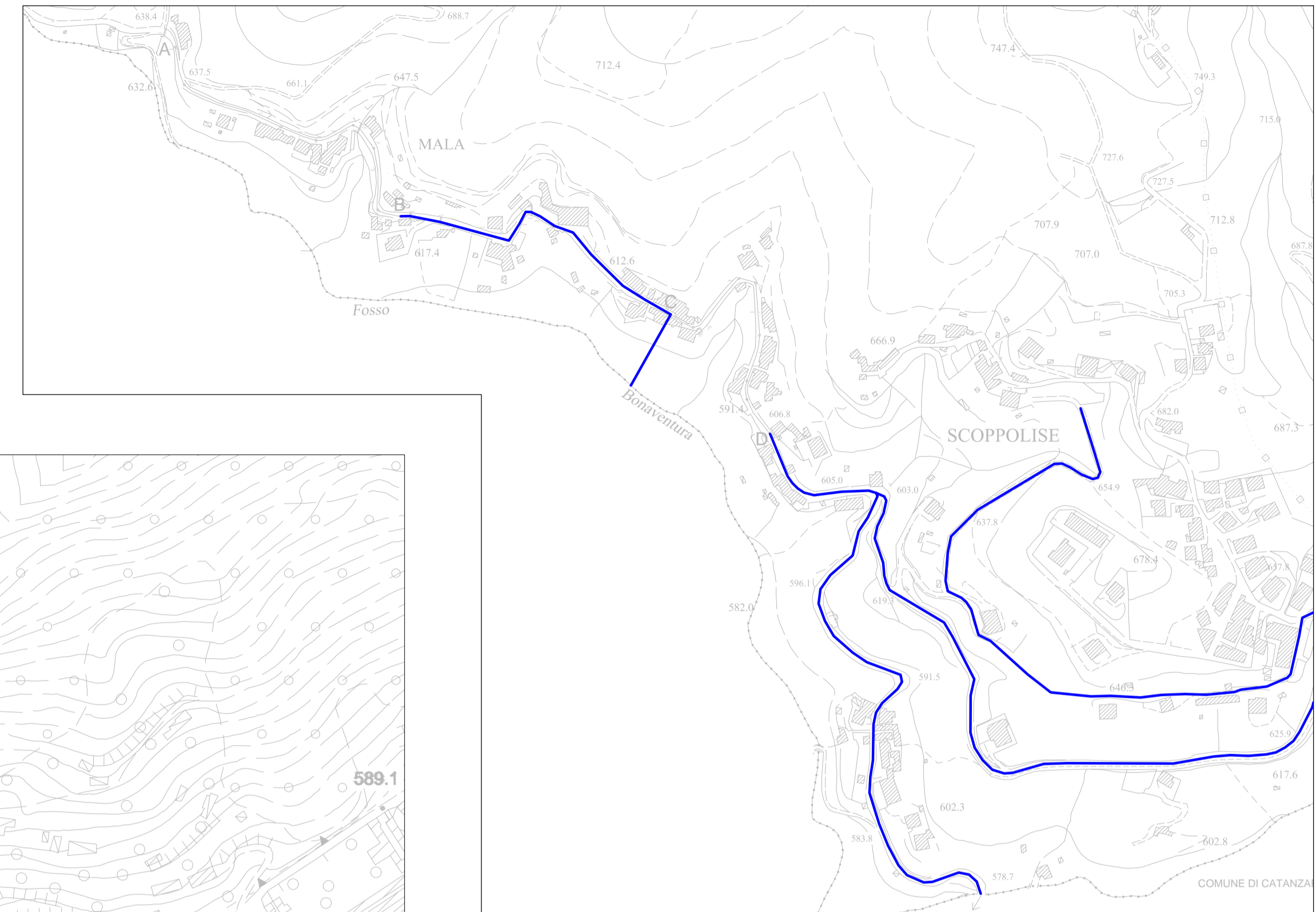
Planimetria Fognatura esistente Località Scoppolise - Frazione Sant'Elia
