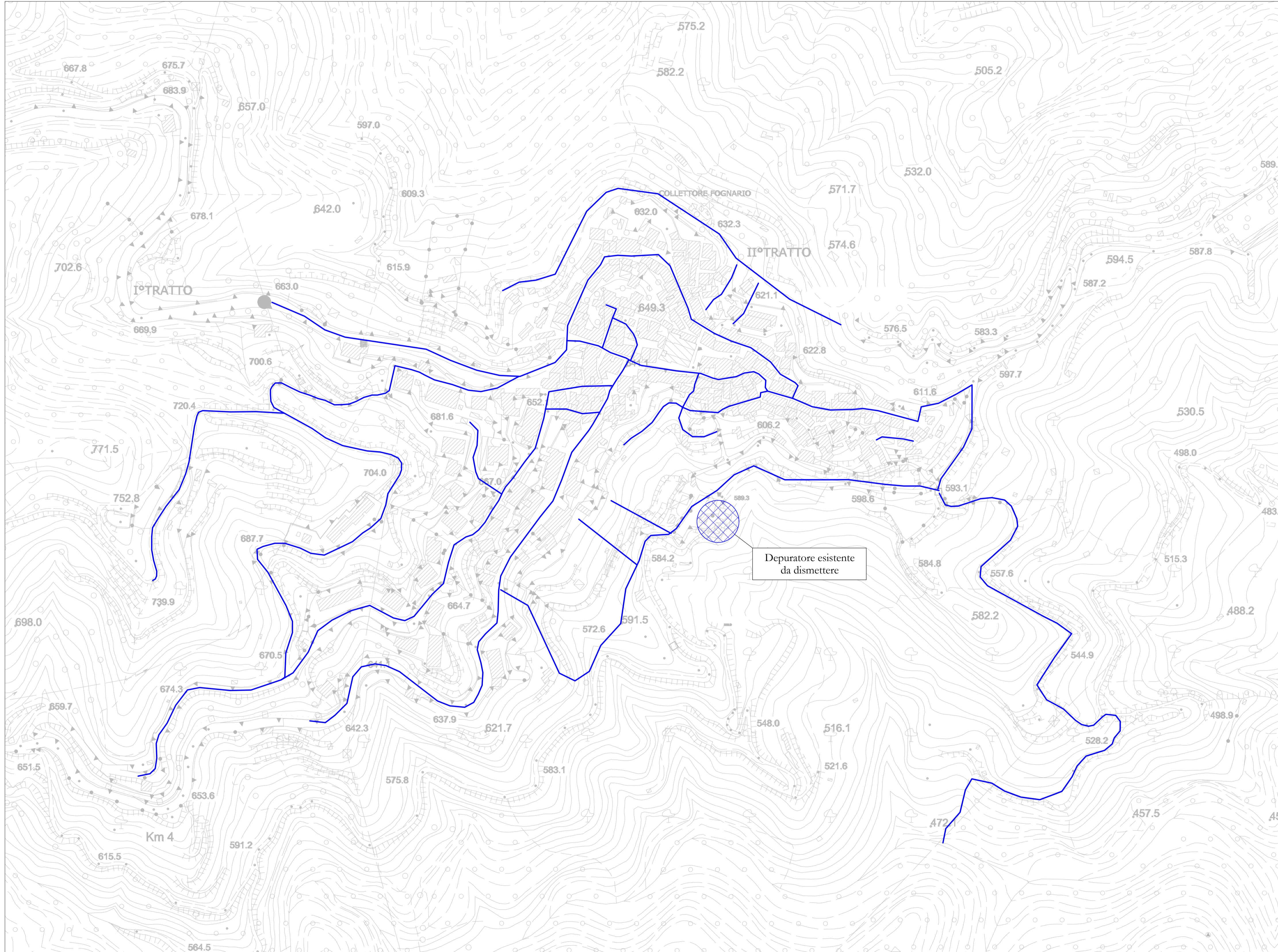
Planimetria Fognatura esistente Pentone Centro
